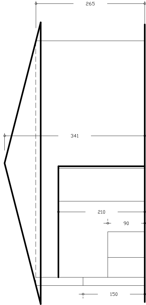
FACHADA LATERAL - DIREITA
