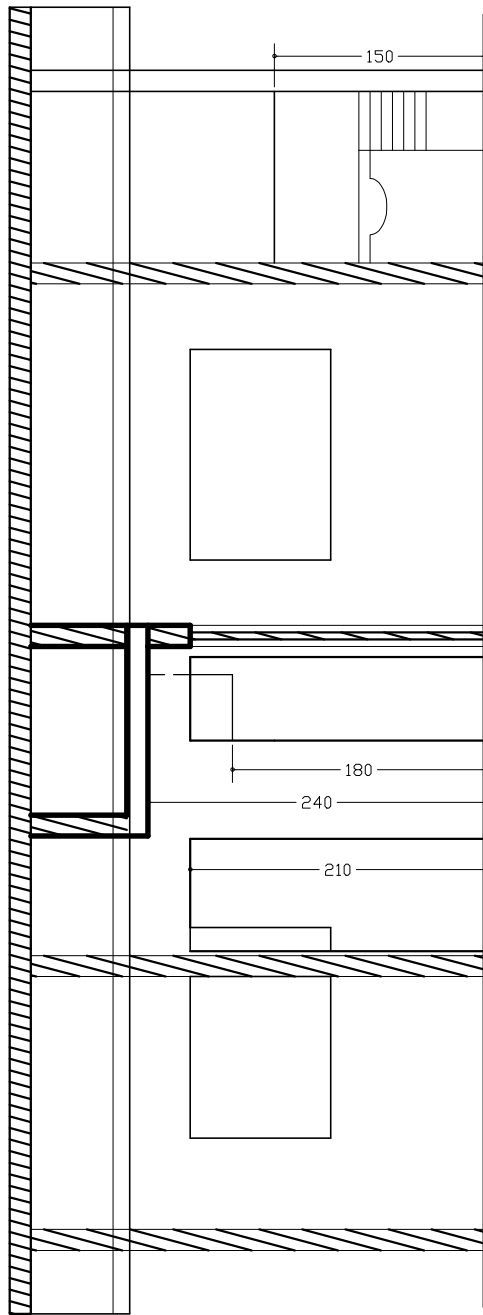
CORTE LONGITUDINAL - CC'
