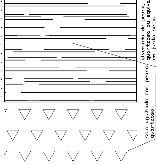
DETALHE DE ALICERCE e CALÇADA
