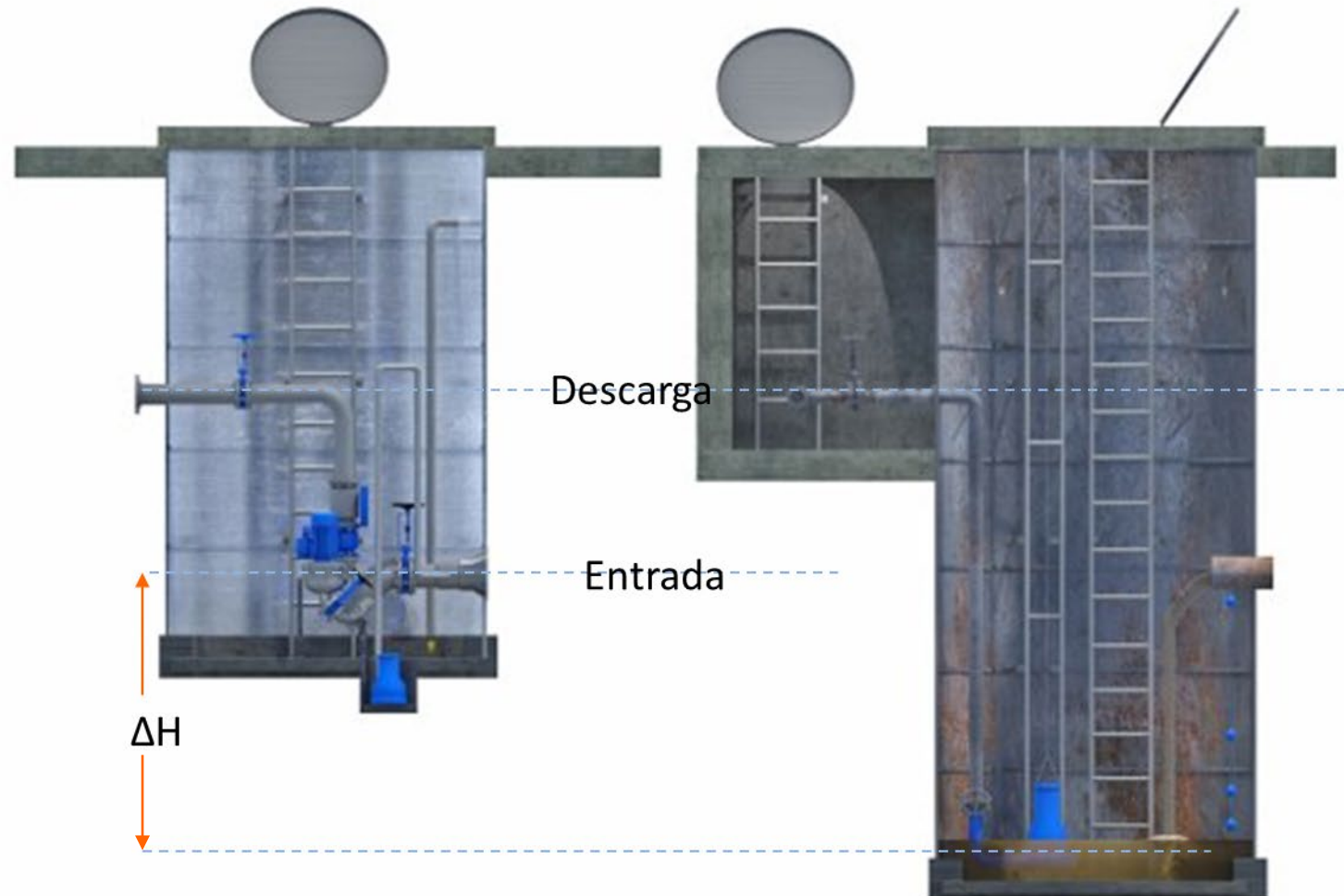
Instalação com Booster de esgoto
