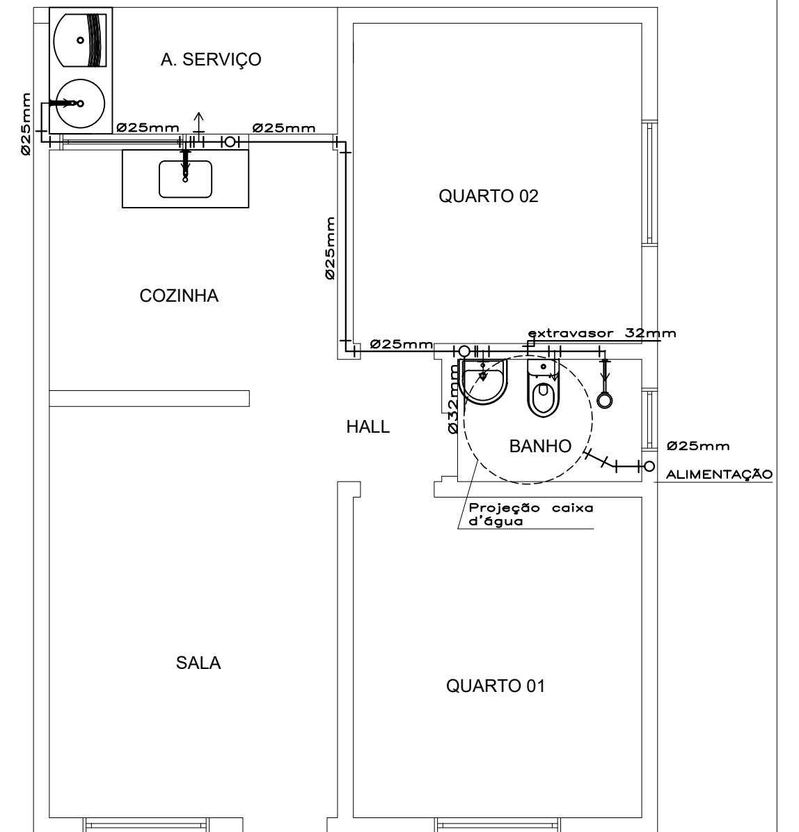
PLANTA BAIXA - REDE DE ÁGUA FRIA
