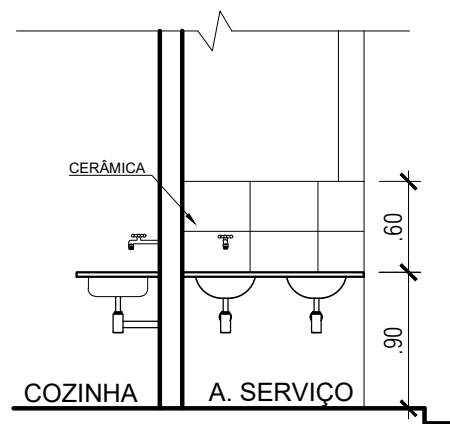
Dets. painel cerâmico cozinha e serviço Esc.: 1/50
