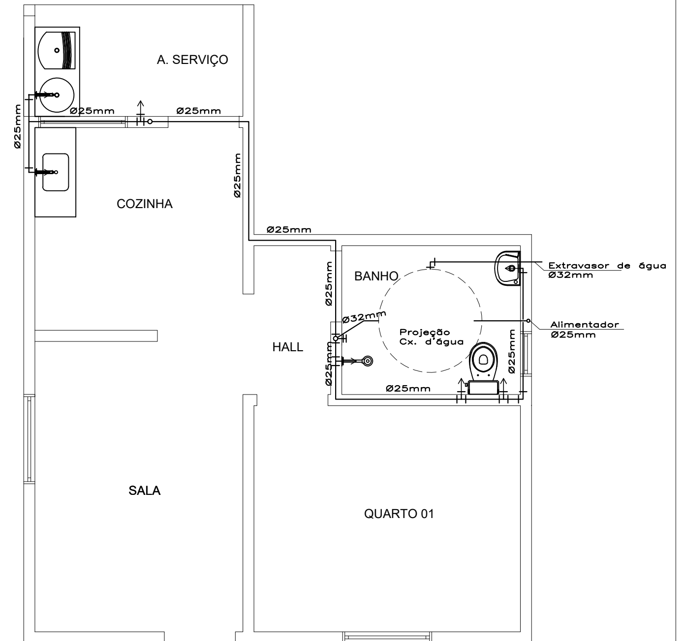
PLANTA BAIXA - REDE DE ÁGUA FRIA
