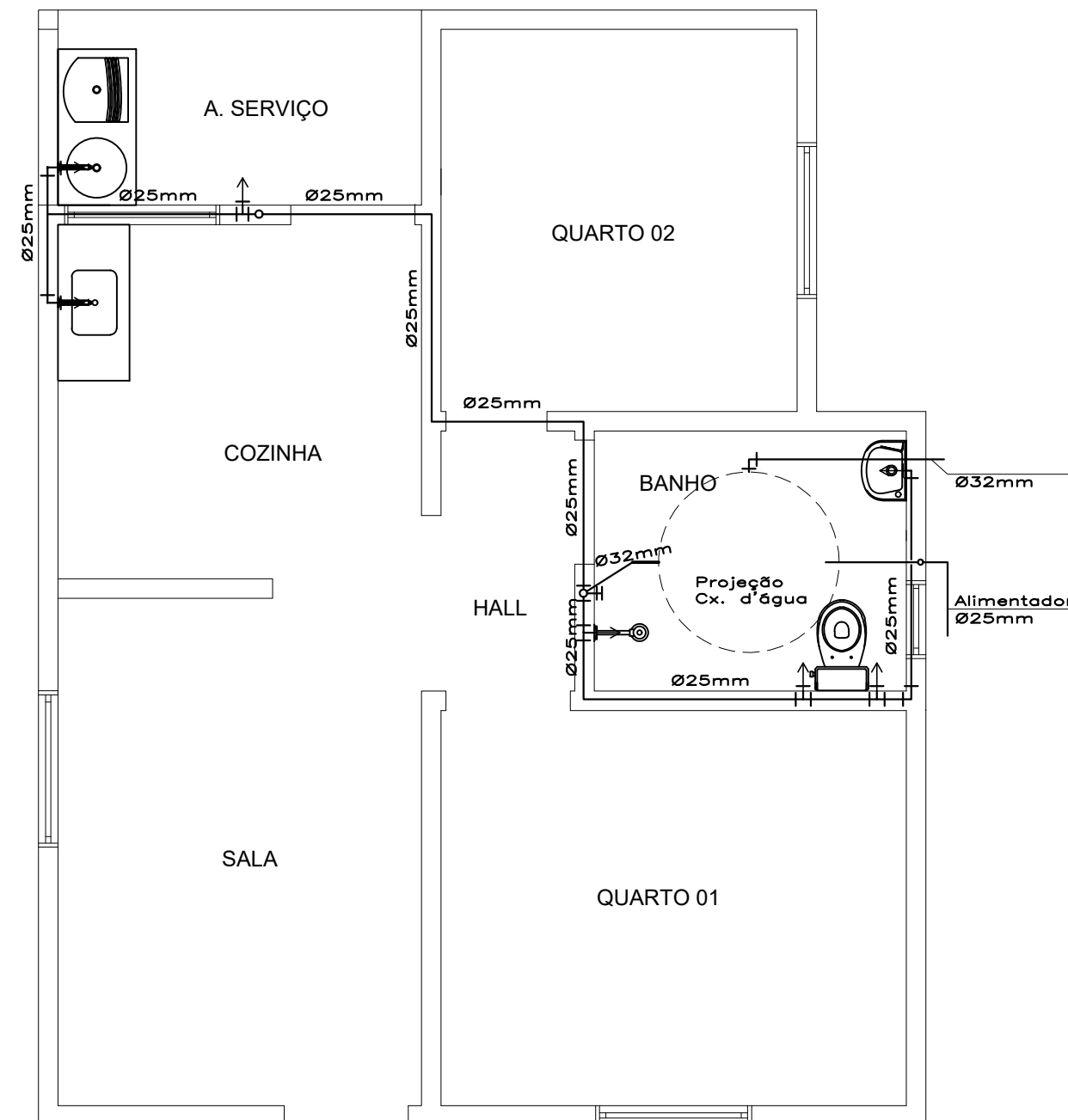
PLANTA BAIXA - REDE DE ÁGUA FRIA
