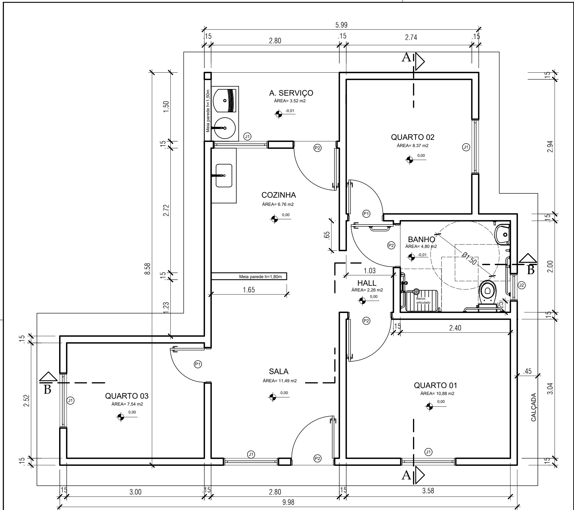
Planta baixa A=64,85m 2 Esc.: 1/50
