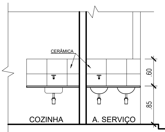
Det. painel cerâmico cozinha e serviço
