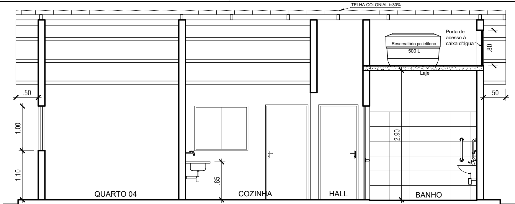
Corte BB
